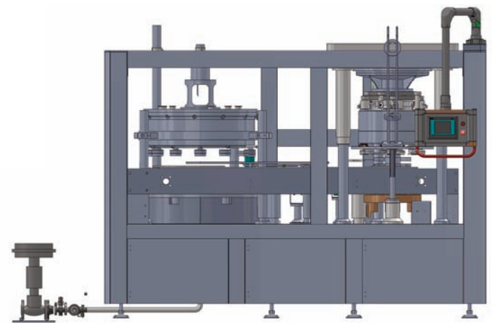
CRAFTBLOC 12/4-100 CPM FILLER/SEAMER
